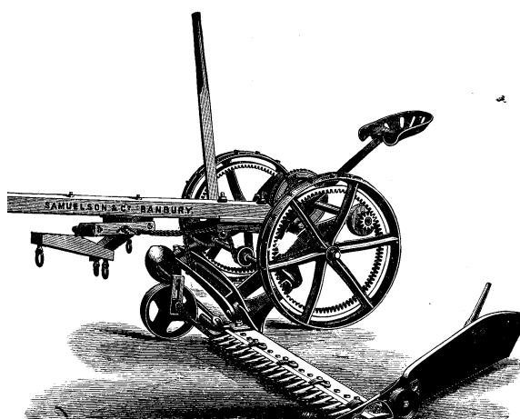
Maaimachine, te trekken door een paard, gebruikt voor het maaien van hooigras en graan. Gebruikt in de eerste helft van de 20 e eeuw.
